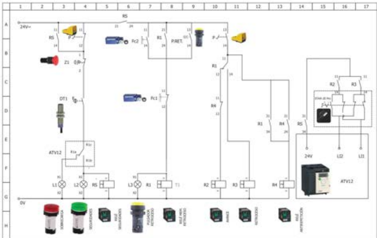
Author: SMA S.A. STAR MONOFÁSICA:Esquema de mando / STAR 1 PHASE:Control scheme / STAR MONOPHASE:Schéma de contrôle Date: 03/05/2023 Folio: 3/4
