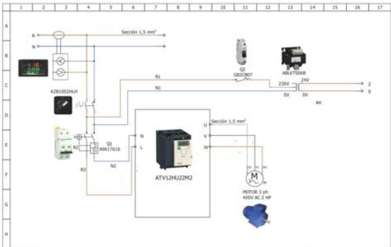
Author: SMA S.A. STAR MONOFÁSICA:Esquema de fuerza / STAR 1 PHASE:Power scheme / STAR MONOPHASE:Schéma de puissance Date: 03/05/2023 Folio: 4/4
