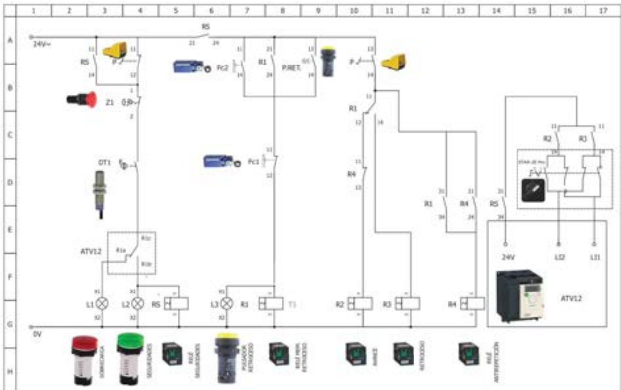
Author: SPM S.A. STAR MONOFÁSICA:Esquema de mando / STAR 1 PHASE:Control scheme / STAR MONOPHASE:Schéma de contrôle Date: 03/05/2023 Hoja: 3/4
